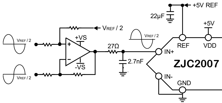
图 31. 双运放实现全差分转单极性伪差分
