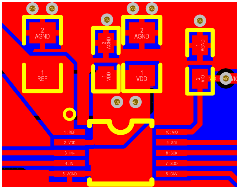
图 48. ZJC2007 的示例布局布线
