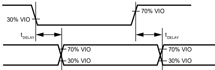
图 6. 时序的逻辑电平
