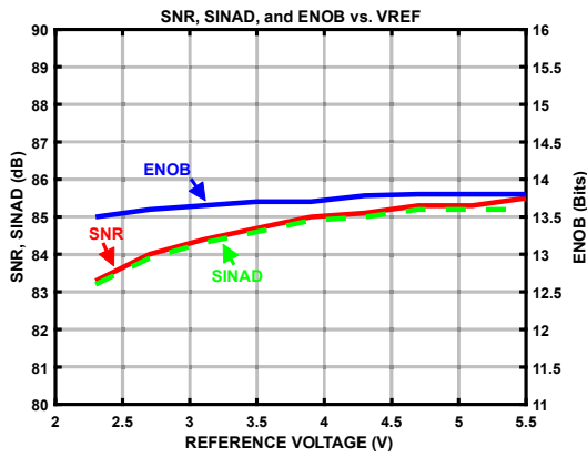
图 13. SNR, SINAD 和 ENOB 与基准电压的关系
