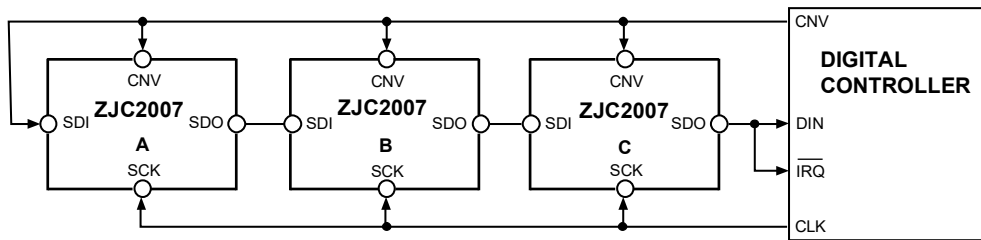
图 46. 链模式(有繁忙指示)连接图
