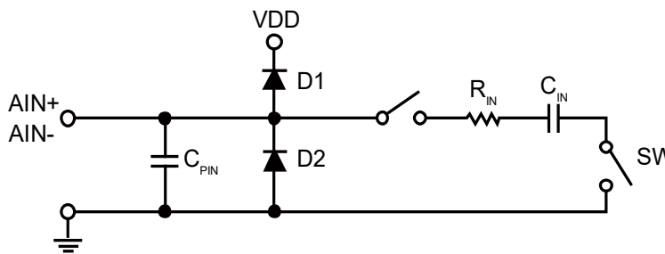
图 28. 两个二极管 D1 和 D2 为模拟输入提供 ESD 保护
