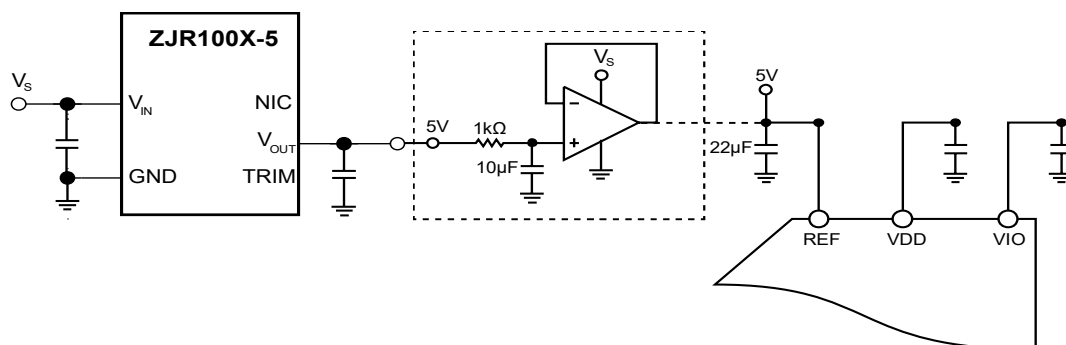
图 33. ZJC2007 参考引脚驱动
