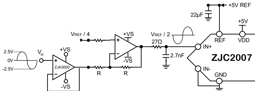
图 32. 双运放实现双极性转单极性伪差分
