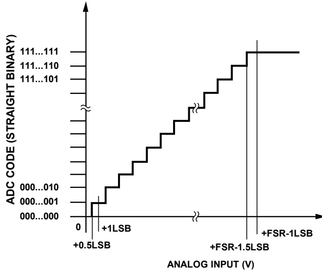
图 26. ADC 理想传递函数
