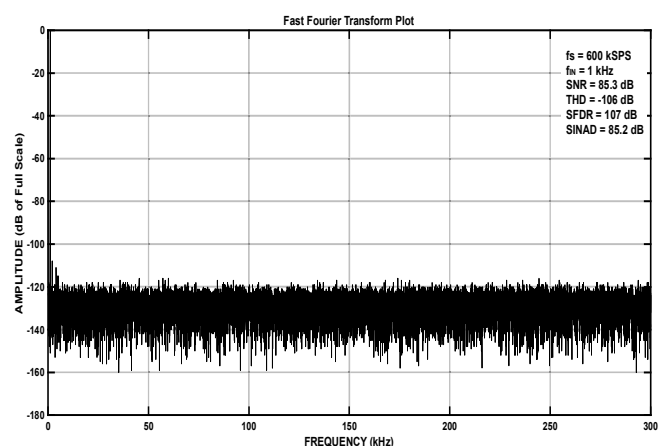
图 2. 交流特性
