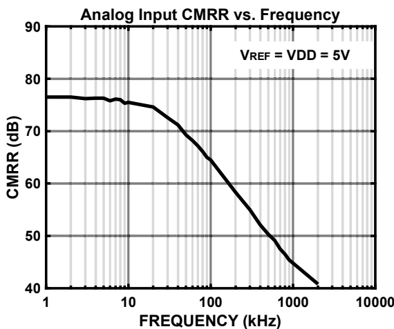
图 29. 模拟输入 CMRR 与频率的关系
