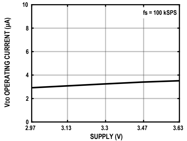
图20. VIO 工作电流与电源电压的关系
