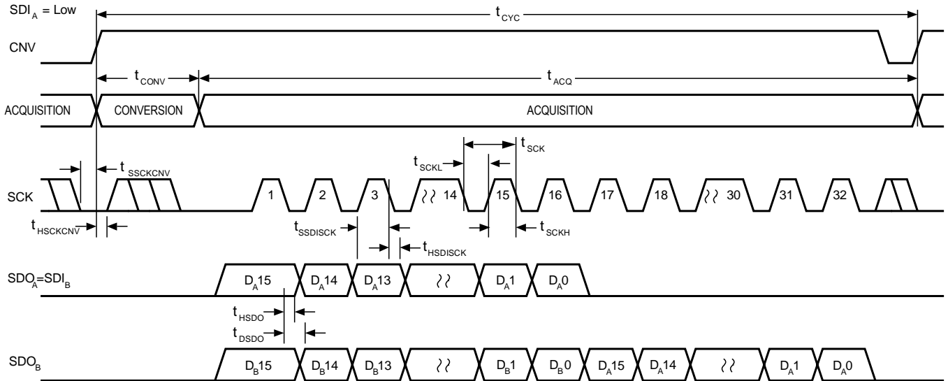
图45. 链模式 (无繁忙指示) 串行接口时序
