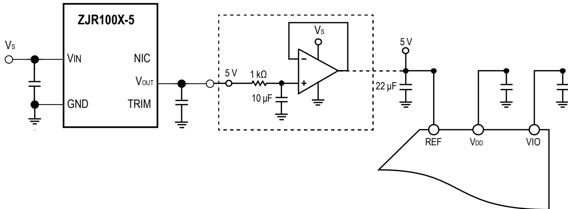
图33. ZJC2003 参考引脚驱动
