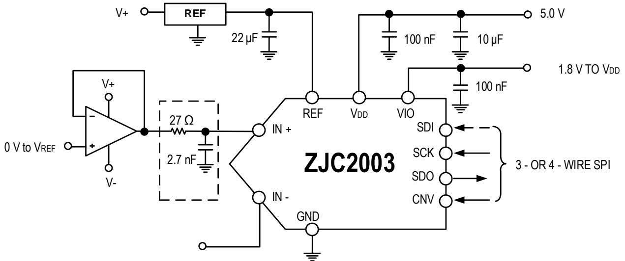
图27. 采用多路电源的应用电路
