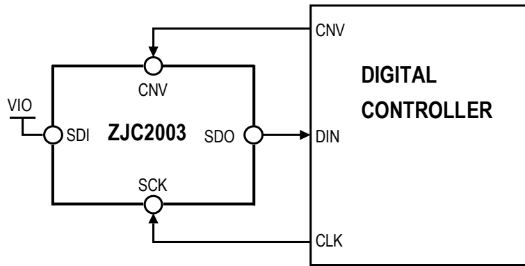
图36. 片选模式 (三线式无繁忙指示) 连接图
