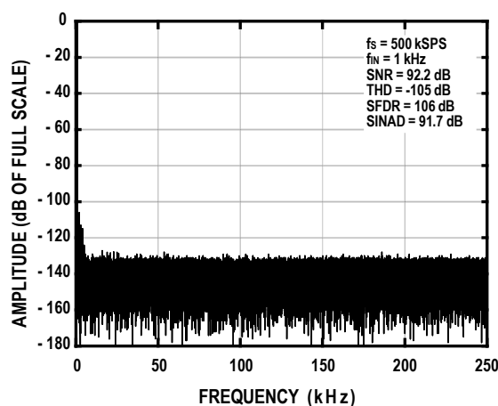
图2. 交流特性
