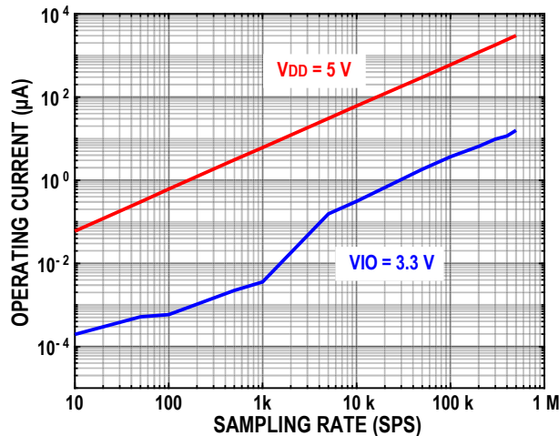
图35. 工作电流与采样速率的关系
