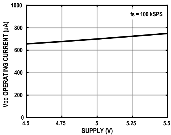
图19. VDD 工作电流与电源电压的关系
