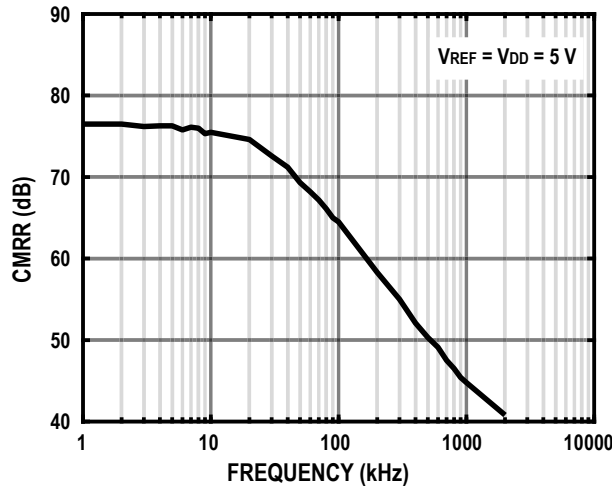
图29. 模拟输入 CMRR 与频率的关系
