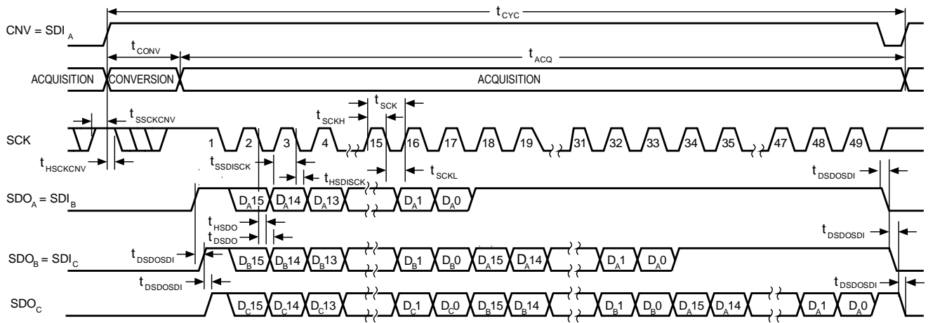
图47. 链模式 (有繁忙指示) 串行接口时序
