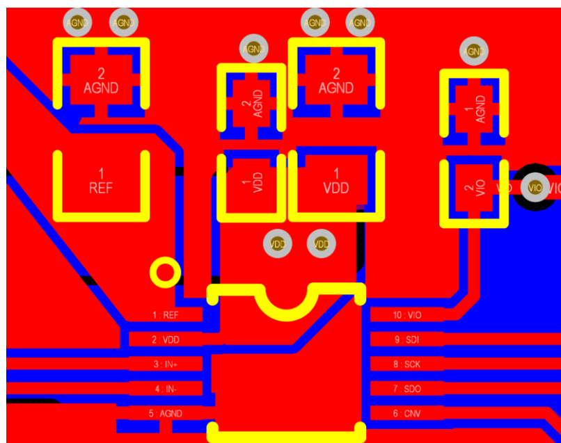
图48. ZJC2003 的示例布局布线
