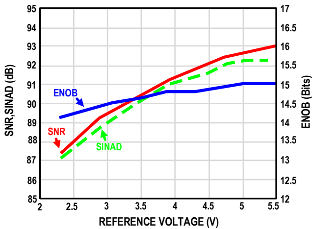
图13. SINAD 和 ENOB 与基准电压的关系
