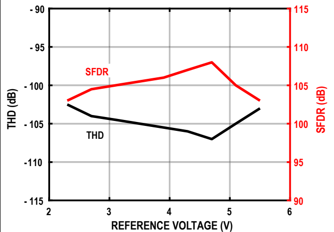
图14. THD, SFDR 与基准电压的关系
