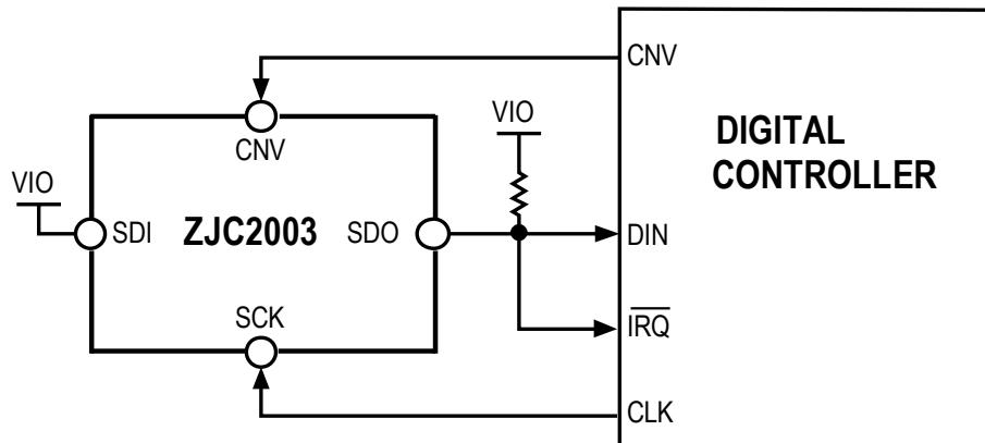
图38. 片选模式 (三线式有繁忙指示) 连接图
