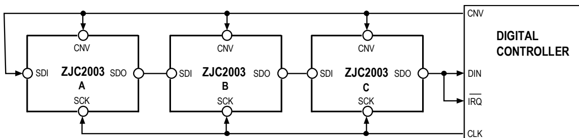
图46. 链模式 (有繁忙指示) 连接图
