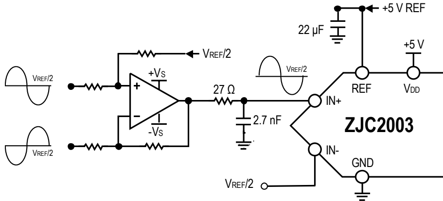
图31. 双运放实现全差分转双极性伪差分
