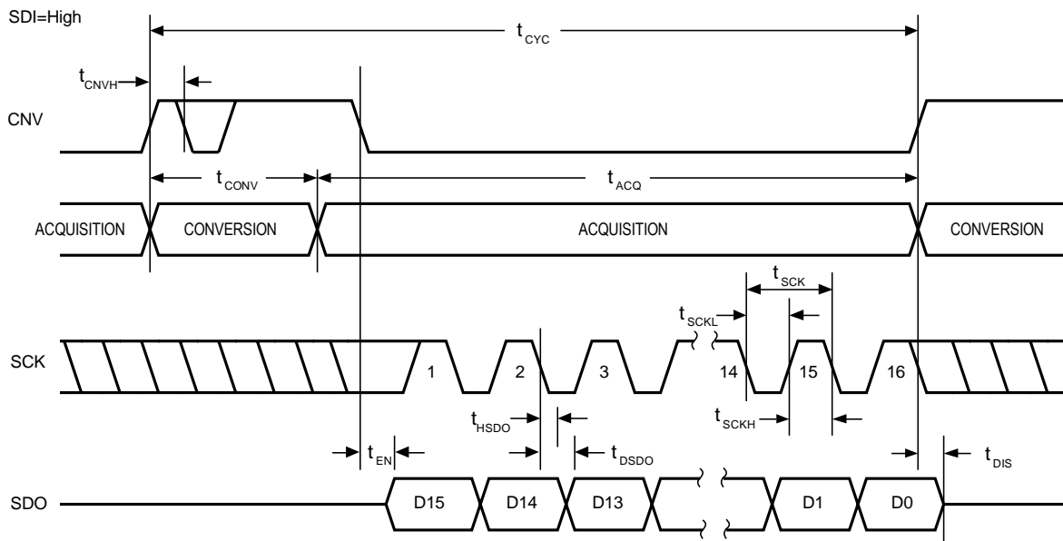
图37. 片选模式 (三线式无繁忙指示) 串行接口时序
