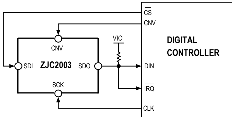
图42. 片选模式 (四线式有繁忙指示) 连接图
