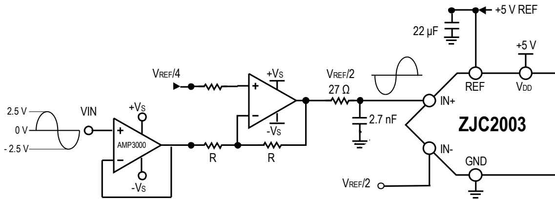
图32. 高输入阻抗双极性单端转双极性伪差分
