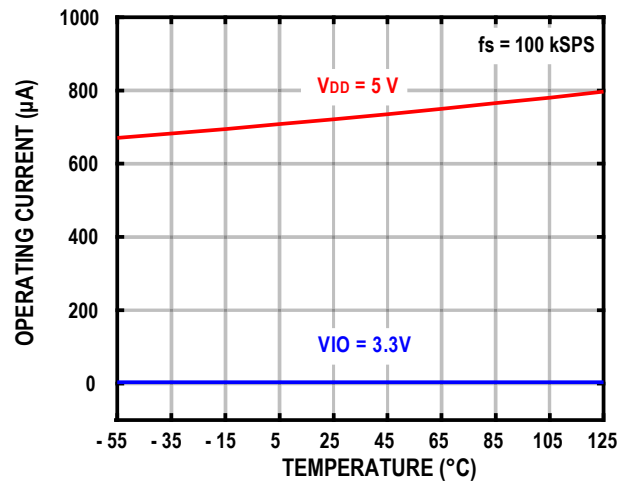
图24. 工作电流与温度的关系
