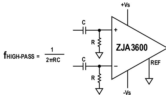
图32. ZJA3600 的交流耦合接法
