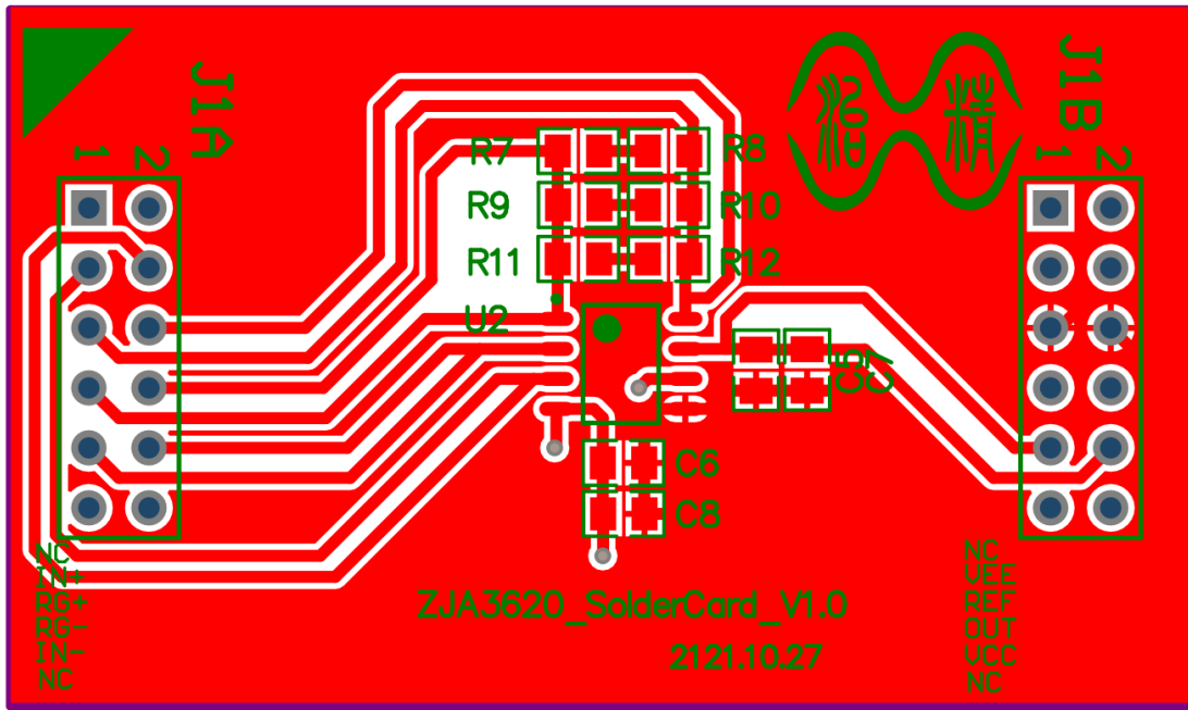
图38. ZJA3620/3600 评估板 PCB 顶层设计
