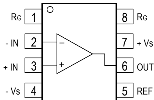
图1. ZJA3600 管脚排列图
