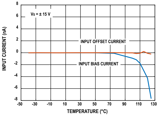
图8. 输入偏置电流 I BIAS 和失调电流 I OS 与温度的关系
