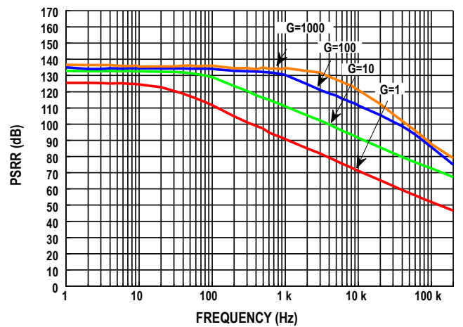
图11. 正 PSRR 与频率的关系, RTI (G = 1 至 1000)
