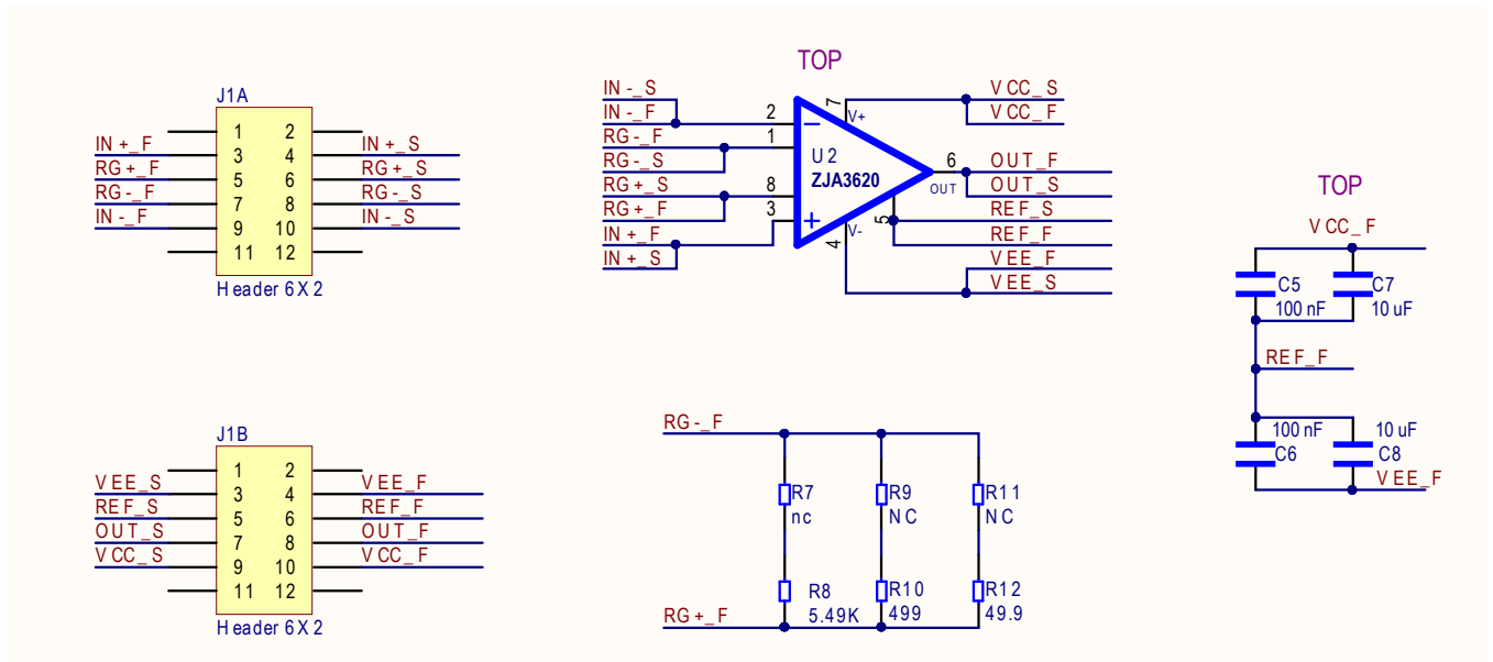
图37. ZJA3620/3600 评估板原理图
