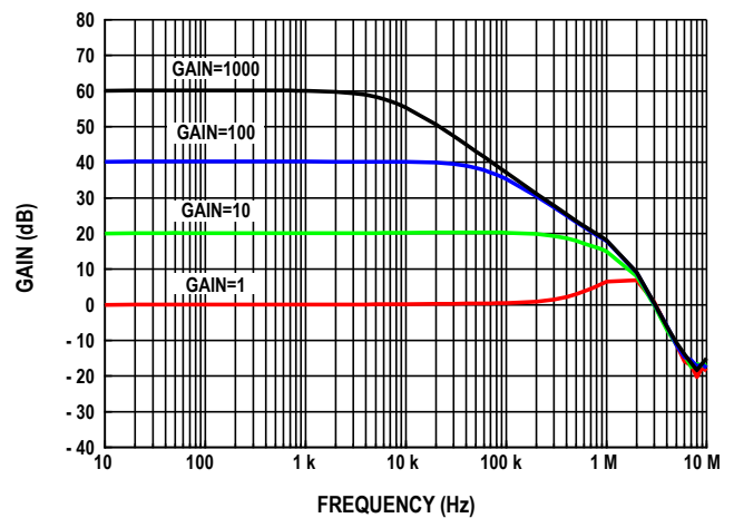
图13. 增益与频率的关系
