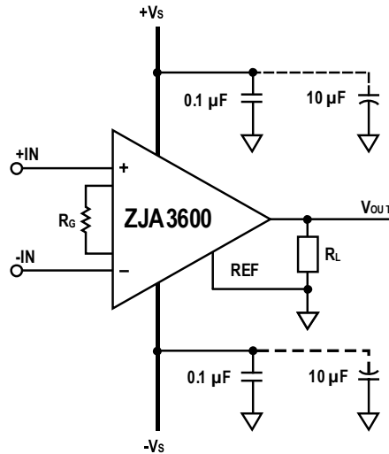
图33. ZJA3600 电源去耦示意图
