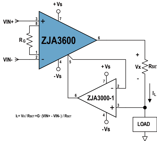
图35. 用 ZJA3600 构建精密电流源
