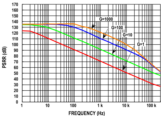
图12. 负 PSRR 与频率的关系, RTI (G = 1 至 1000)
