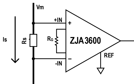
图36. ZJA3600 用于精密电流检测
