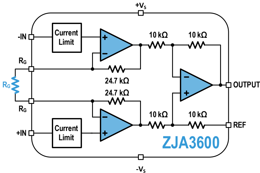
图29. ZJA3600 简化的示意图
