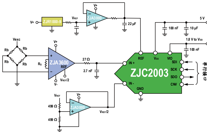
图34. 桥式电路与 ZJA3600 接口
