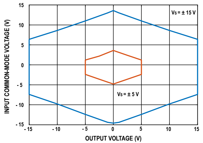
图9. 输入共模电压范围与输出电压的关系 (G = 1)
