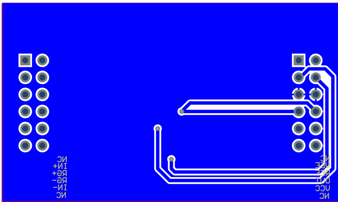
图39. ZJA3620/3600 评估板 PCB 底层设计
