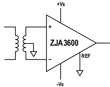
图31. ZJA3600 与变压器的连接
