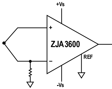
图30. ZJA3600 与热电偶的连接
