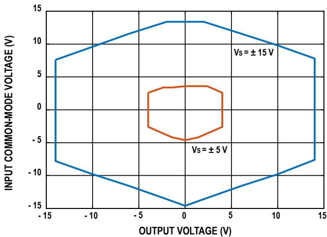
图10. 输入共模电压范围与输出电压的关系 (G = 100)
