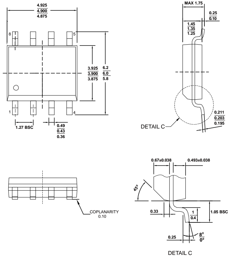
图40. SOIC-8 封装尺寸图 (单位: 毫米)
