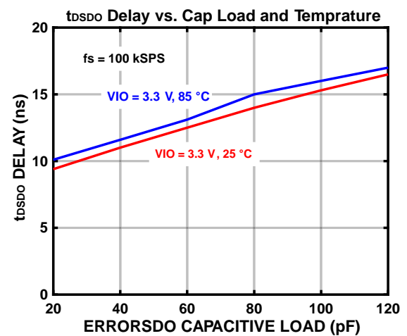
图23. tSDO 延时 vs 负载电容和电压
