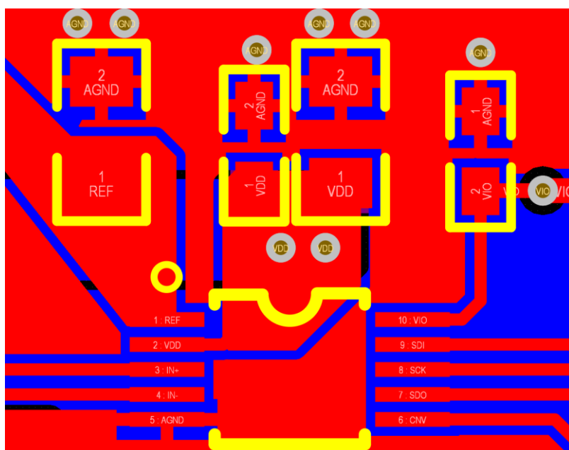
图48. ZJC2014 的示例布局布线
