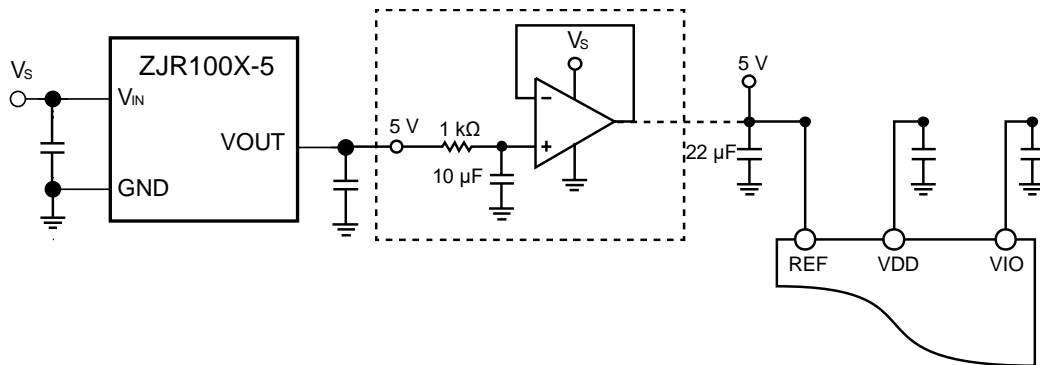
图33. ZJC2014 参考引脚驱动
