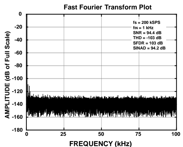
图2. 交流特性
