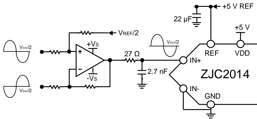
图31. 双运放实现全差分转单极性伪差分
