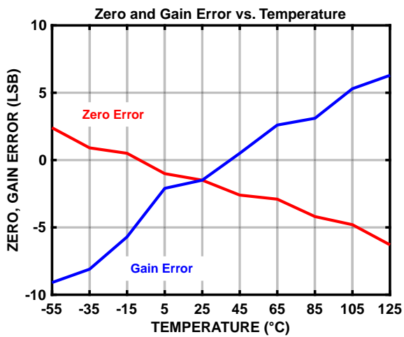
图21. 零输入，增益误差与温度的关系
