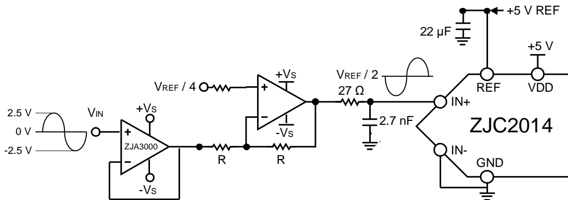
图32. 双运放实现双极性单端转单极性伪差分
